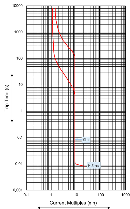
DN3B MCCB
