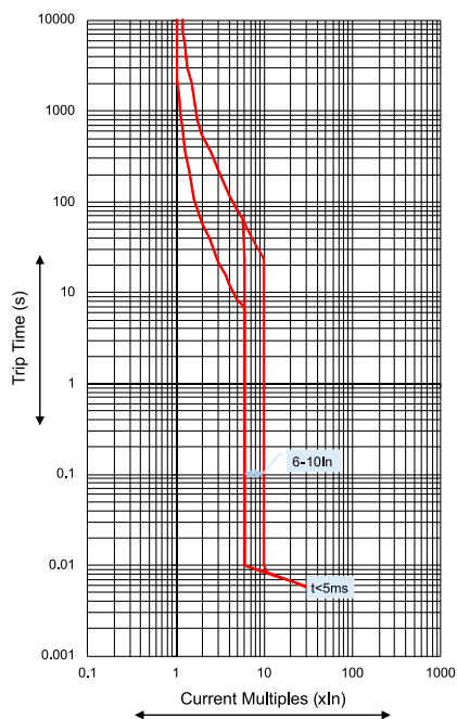
DN2 MCCB
