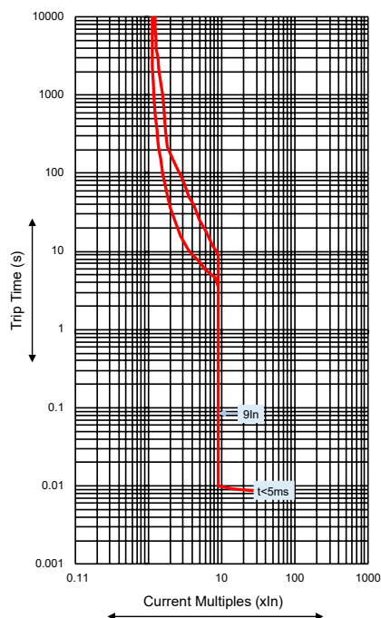
DN1 MCCB
