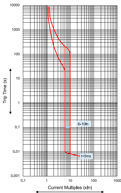
DN3 MCCB
