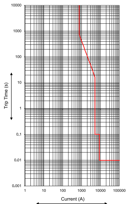
DN3T MTX3.0
